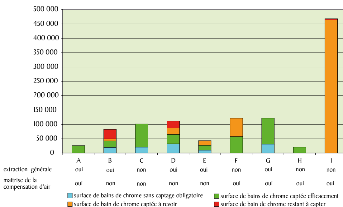
Graphique 13 - Représentation graphique des surfaces de baignoires de chrome en \text{cm}^2 en fonction du captage des baignoires existantes comparées à ceux recommandés dans le guide de ventilation du traitement de surface
