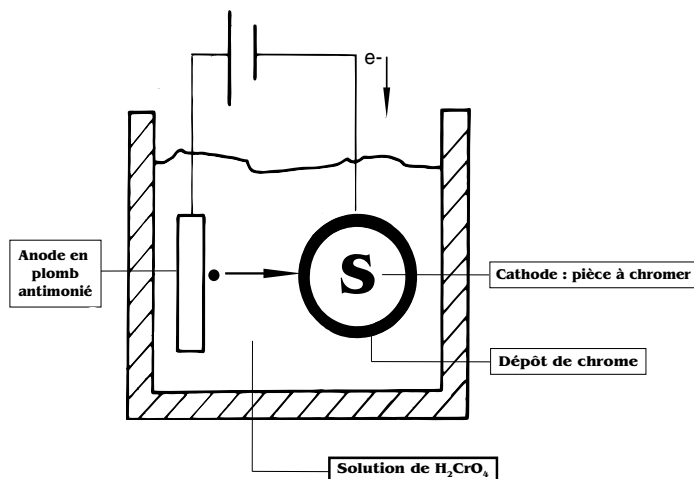
Graphique 9 - Principe de réaction conduisant au dépôt de chrome métallique
