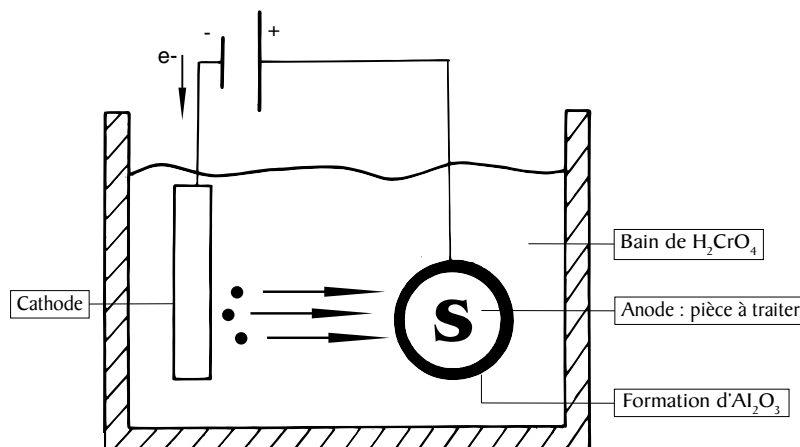
Graphique 10 - Principe de réaction de l'oxydation anodique chromique
