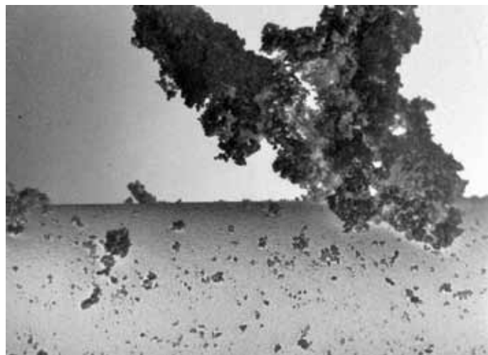
Particules Diesel sur une fibre de 5 µm
